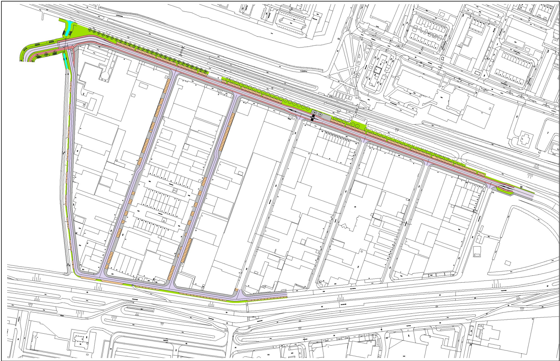
Figuur 1: ontwerptekening opgesteld in samenwerking met de ondernemers.
